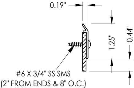
8 DOOR SWEEP NGP 200 N-S
